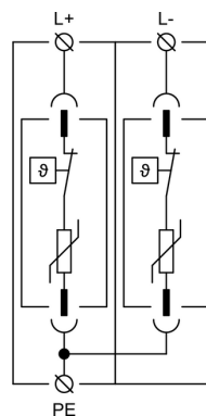
Schemat okablowania wewnętrznego
