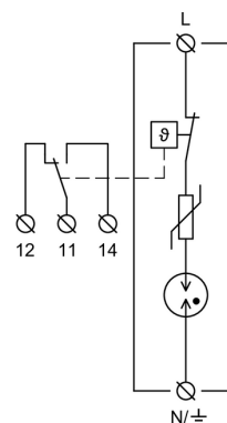
Vnútorná schéma zapojenia
