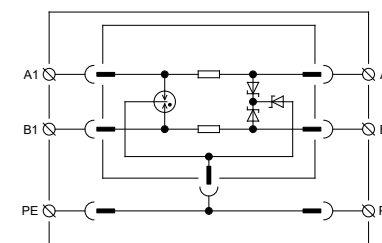
DTNVE M 1/CIB module One pair data transmission Jednopárové datové přenosy
