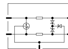
DTNVE M 1/CIB module One pair data transmission Jednopárové datové přenosy
