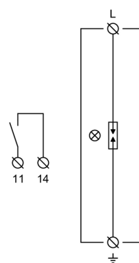
Vnitřní schéma zapojení
