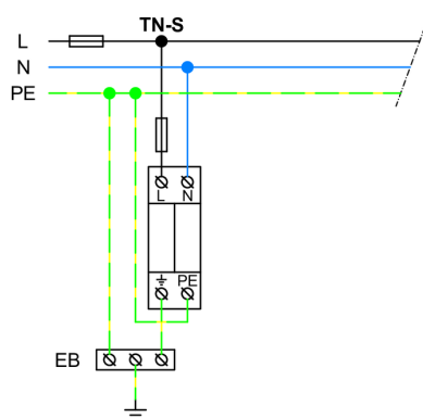
Aplikační schéma zapojení (instalace)
