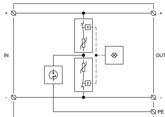
Vnitřní schéma zapojení
