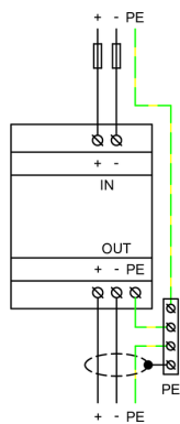
Aplikační schéma zapojení (instalace)
