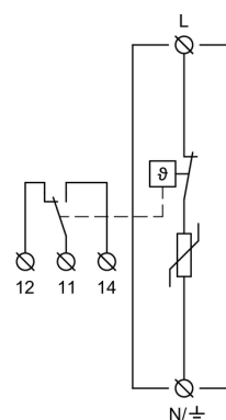
Vnútorná schéma zapojenia
