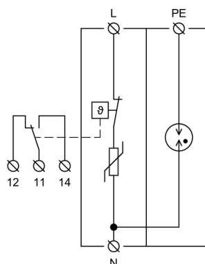
Vnútorná schéma zapojenia
