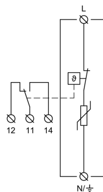
Vnútrotná schéma zapojenia
