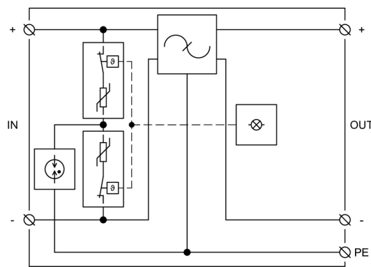
Vnútrotná schéma zapojenia
