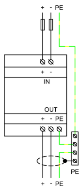
Aplikačná schéma zapojenia (inštalácia)
