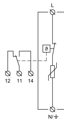
Vnútná schéma zapojenia
