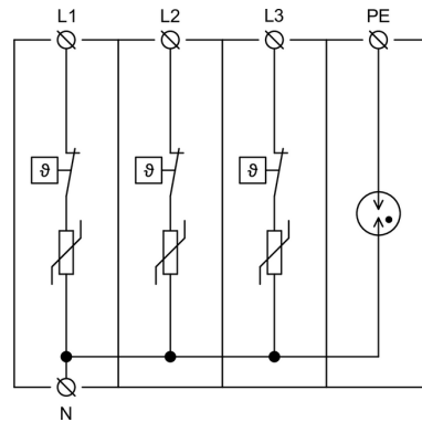
Внутренняя электрическая схема
