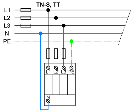
Схема электрических соединений (установка)
